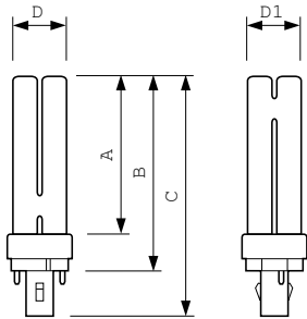
PL-C 13W/830/2P
