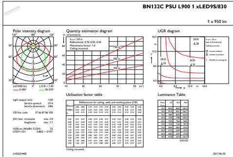
IFGU1_BN132CPSUL9001xLED9S830
